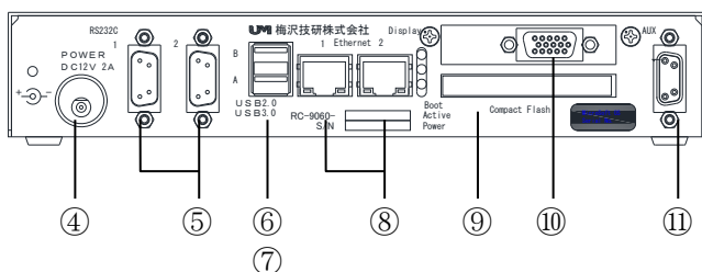
RC-9060-VGA+AUDIO TypeW10
